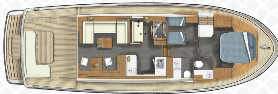
Aufteilung Linssen 45 SL Sedan
